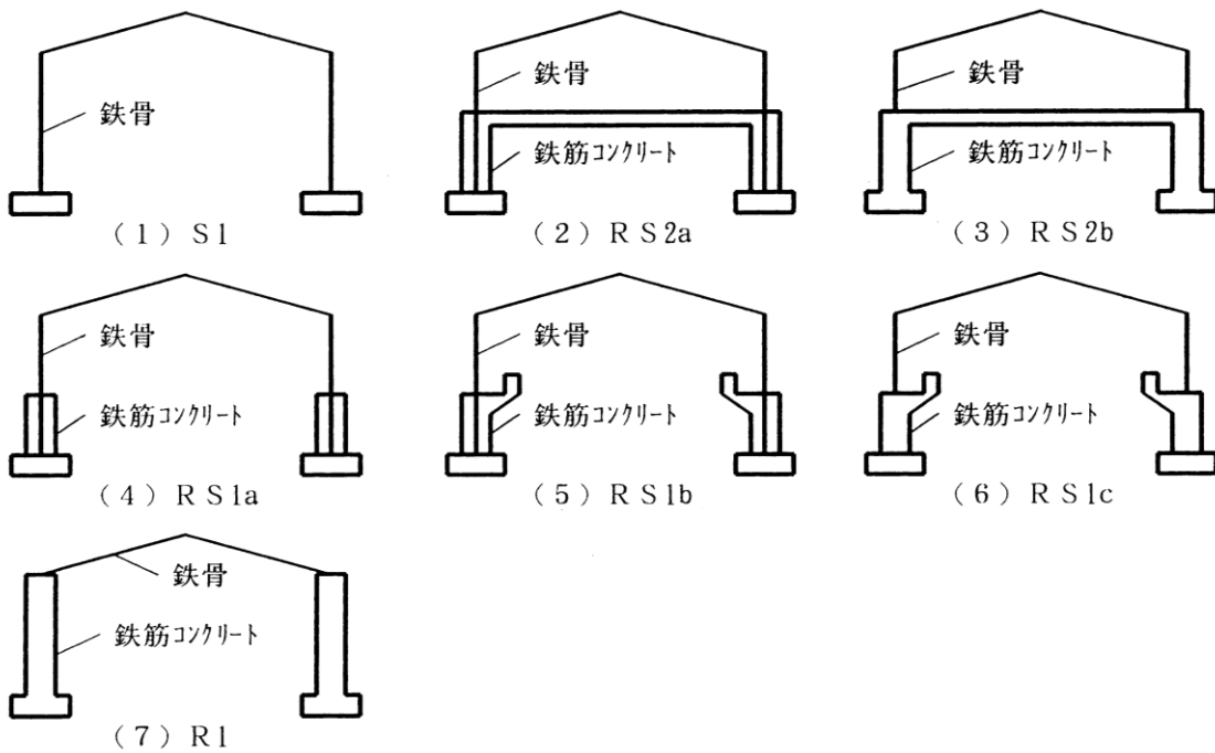
図-2 架構種別
