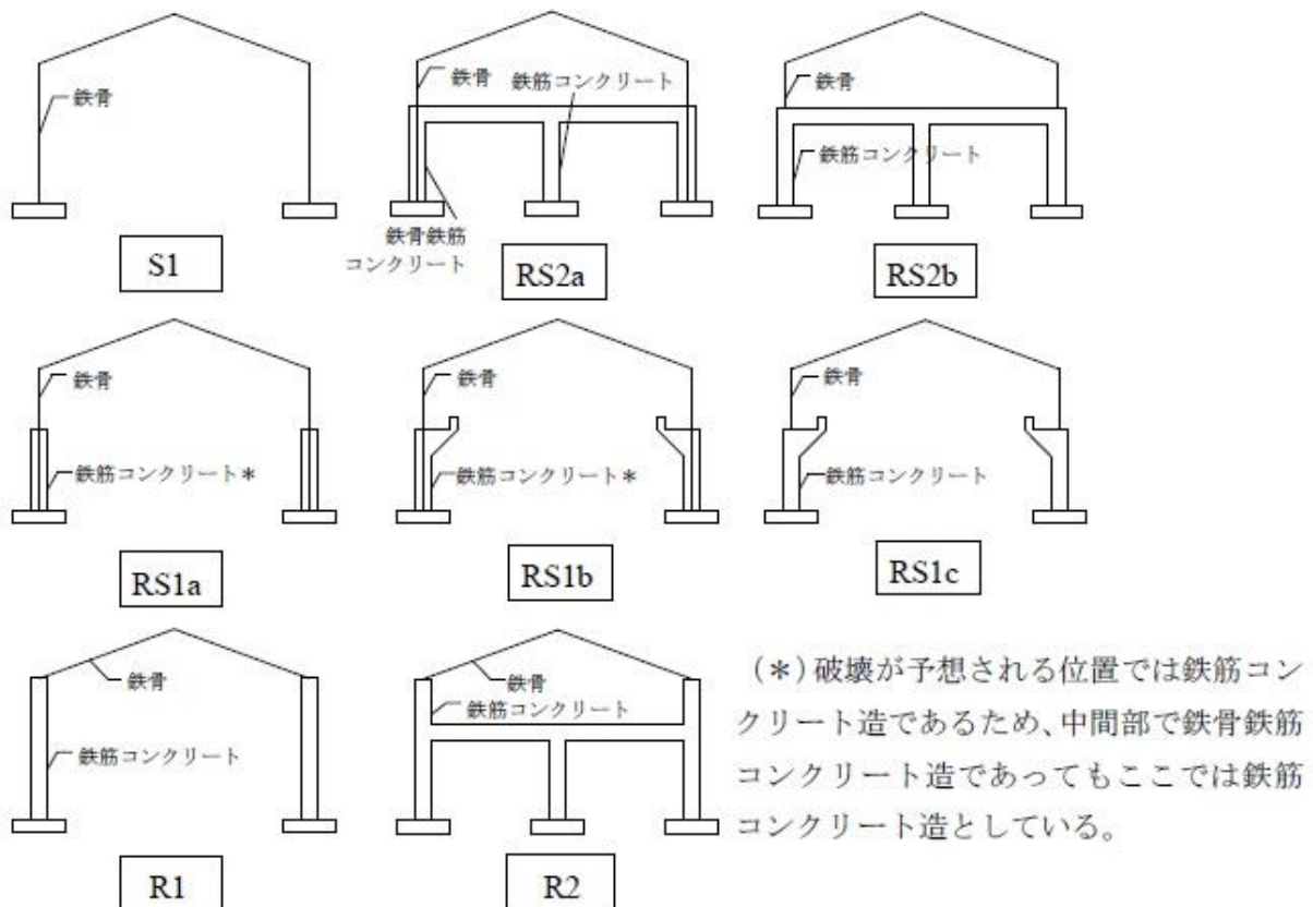
図-2 架構種別
