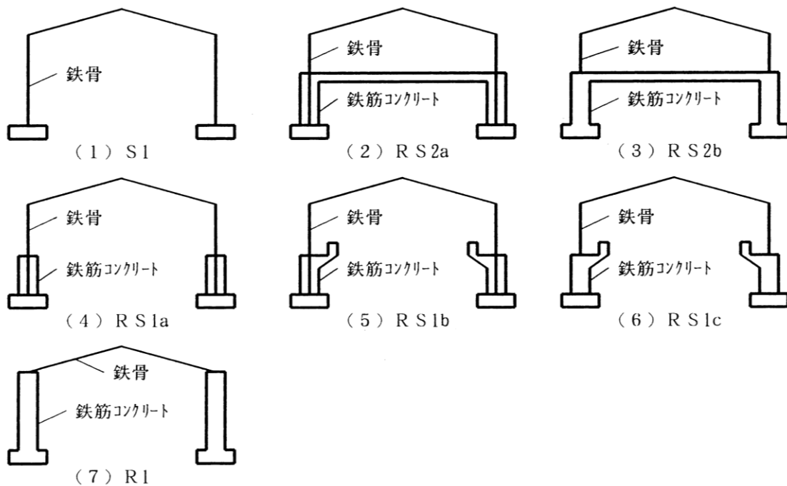
図-2 架構種別
